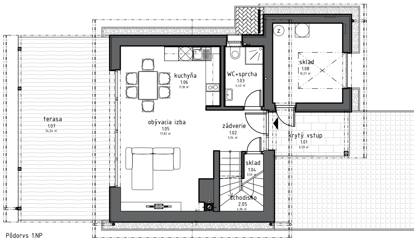
Pôdorys 1.NP
